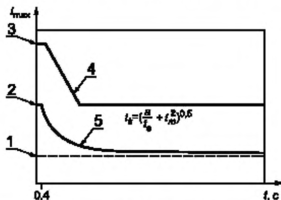
1 — абсолютный минимум I_{\min} ; 2 — I_k при t_k = 0,4 с; 3 — эффективный ток предварительного подогрева; 4 — максимальный эффективный ток предварительного подогрева в любой момент времени t ; 5 — предел минимального эффективного тока предварительного подогрева за время t_k
