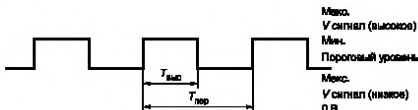
Типичный ШИМ сигнал
