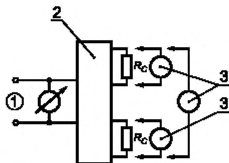
1 — сеть; 2 — испытуемый ПРА; 3 — измерительное устройство
