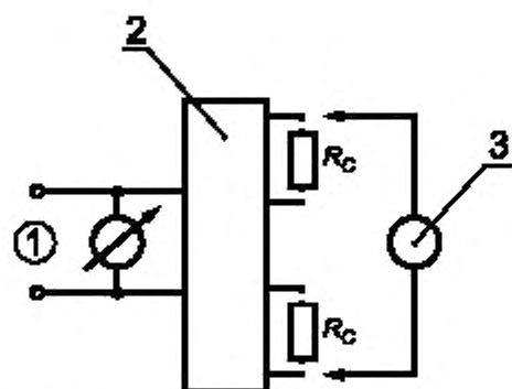
1 — сеть; 2 — испытуемый ПРА; 3 — измерительное устройство
