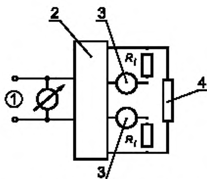
1 — сеть; 2 — испытуемый ПРА; 3 — измерительное устройство; 4 — лампа
