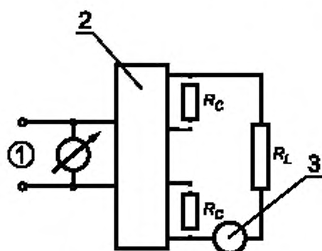
1 — сеть; 2 — испытуемый ПРА; 3 — измерительное устройство
