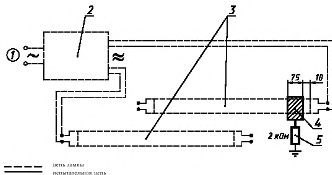
1 — сеть; 2 — высокочастотный ПРА; 3 — лампы; 4 — металлическая фольга; 5 — безындуктивный резистор
