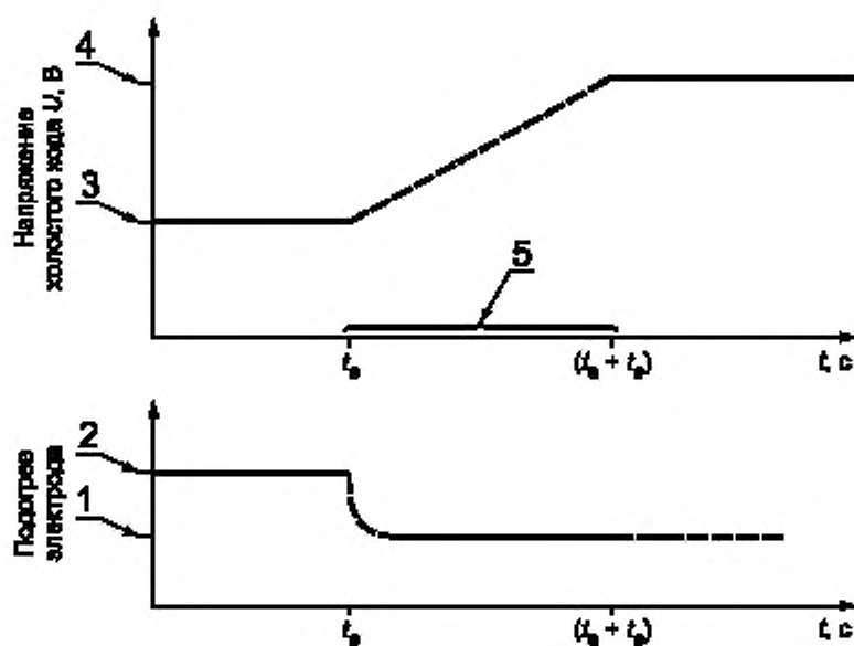
Рисунок В.3.1 — Стартеры, которые прекращают ток предварительного подогрева при повышении напряжения холостого хода
