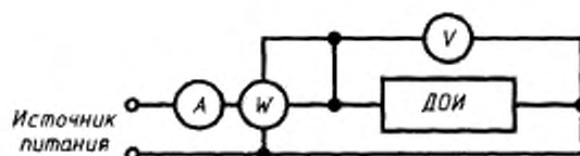
Рисунок 2 — Схема измерения коэффициента мощности
