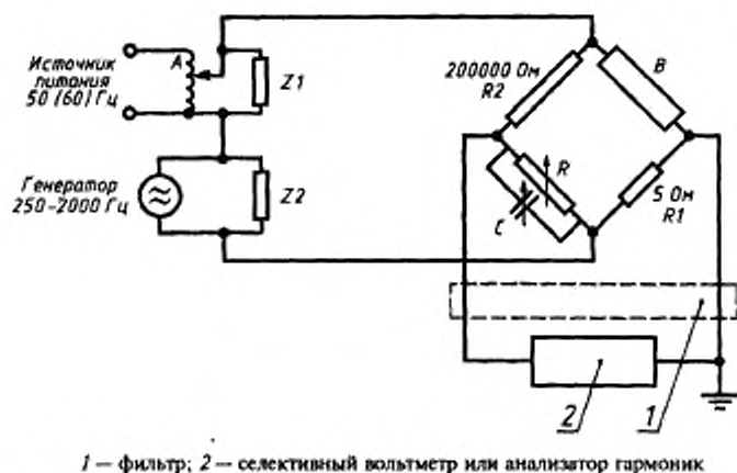
Рисунок 10 — Схема измерения полного сопротивления на звуковых частотах. Способ А
