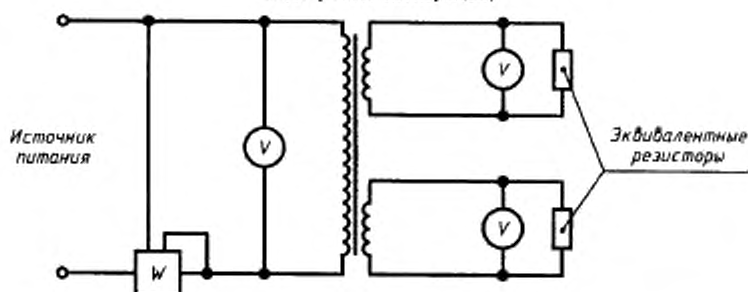
Рисунок 5 — Схема калибровки трансформаторов предварительного подогрева
