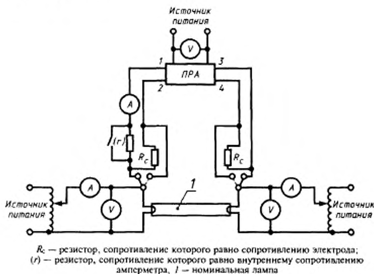
Рисунок 8 — Схема измерения максимального тока во вводах
