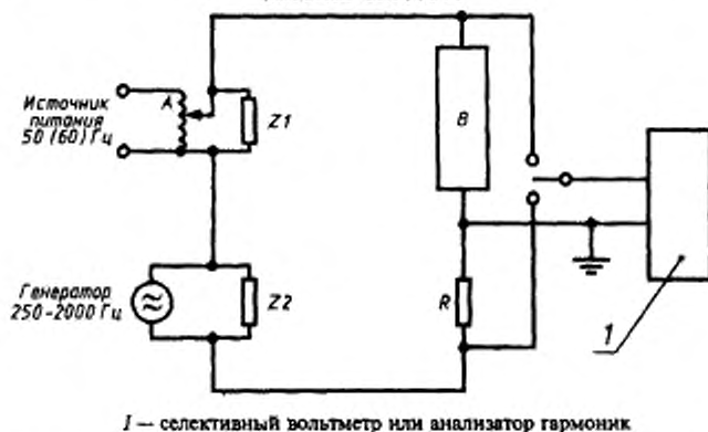
Рисунок 10 — Схема измерения полного сопротивления на звуковых частотах. Способ А
