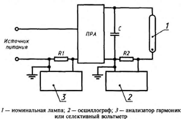
Рисунок 9 — Схема измерения формы кривой тока
