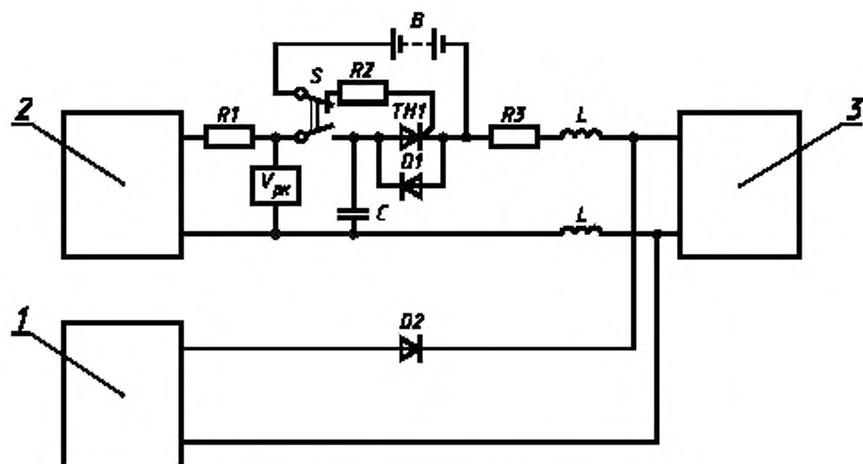
1 — блок питания PSU1; 2 — блок питания PSU2; 3 — испытуемый инвертор
