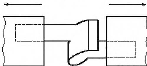
Рисунок 6 — Способ зажима испытуемой пробы в форме брюк
