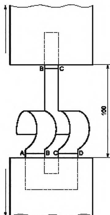
Рисунок 3 — Способ заправки языковой испытуемой пробы
