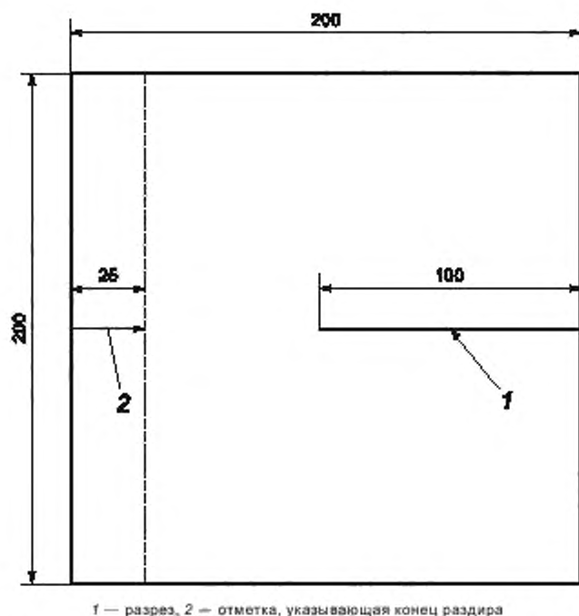
Рисунок В.1 — Испытуемая проба большой ширины в форме брюк
