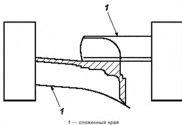
Рисунок В.2 — Способ заправки испытуемой пробы большой ширины в виде броек
