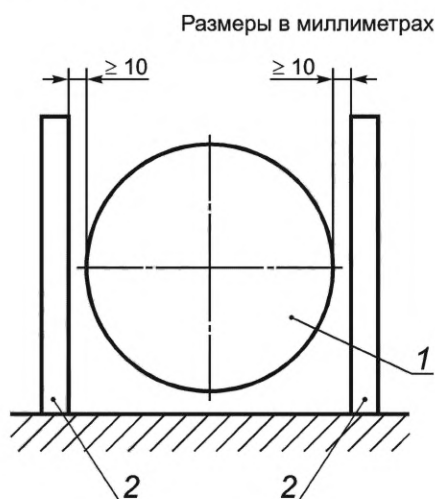
1 — режущее устройство; 2 — испытательный стержень
