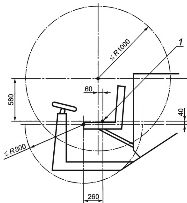
Рисунок 2 — Зоны досягаемости для верхних и нижних конечностей оператора в положении сидя
