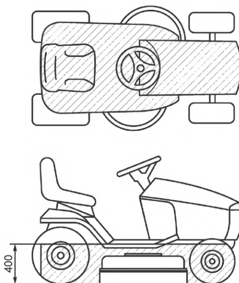
Рисунок В.1 — Пример габаритных размеров рамы для полунавесного режущего устройства
