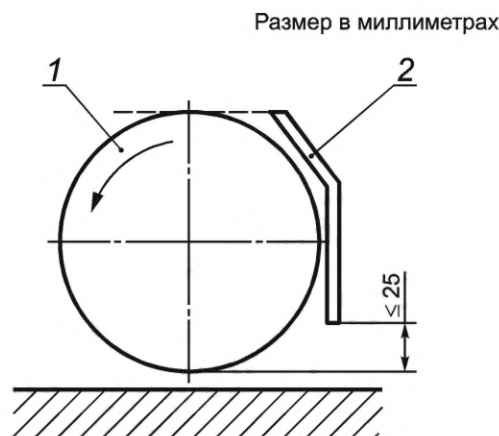
Рисунок 10 — Защитное ограждение режущего устройства, выброс свободный или назад
