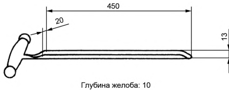
Рисунок А.1 — Щуп для отбора проб (открытый триер)
