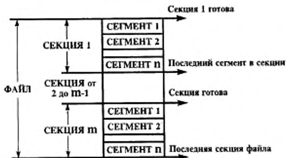
Рисунок 20 — Общее построение файла
