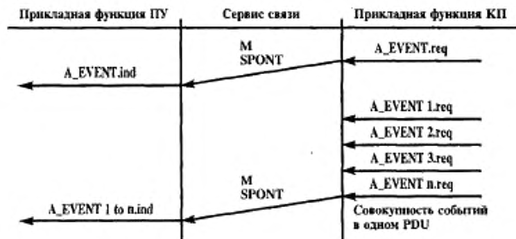
Рисунок 12 — Последовательная процедура сбора данных о событиях
