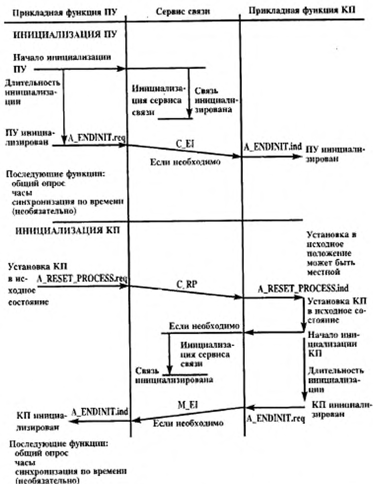
Рисунок 3 — Последовательная процедура — основная процедура инициализации
