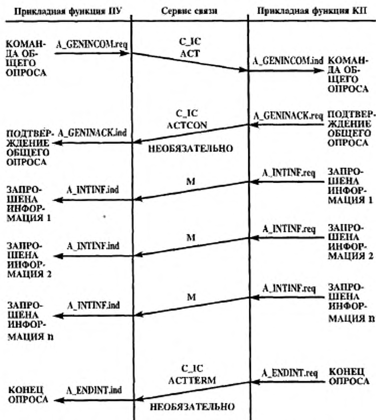
Рисунок 14 — Последовательная процедура — процедура опроса подстанций
