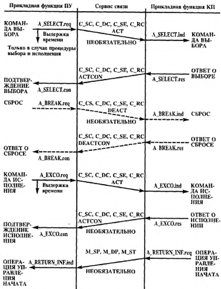
Рисунок 16 — Последовательная процедура — процедура передачи команд, лист 1
