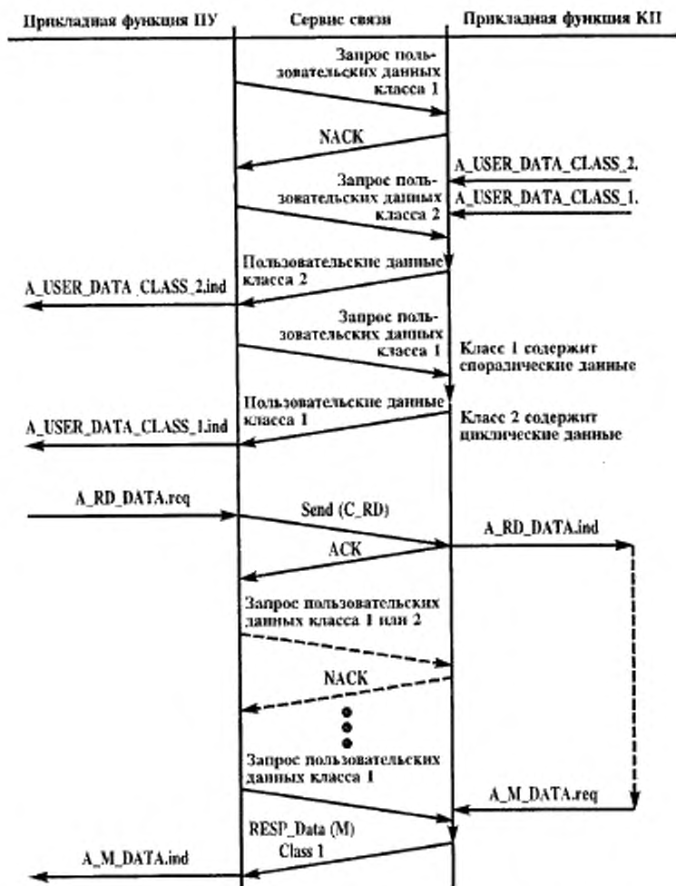
Рисунок 10 — Последовательная процедура — процедура опроса
