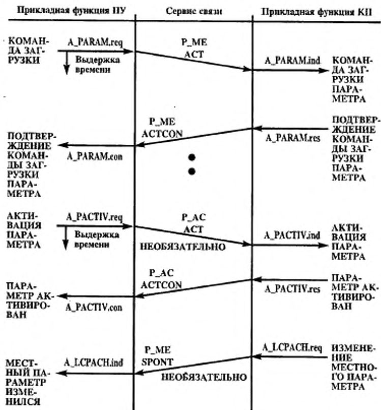
Рисунок 18 — Последовательная процедура — загрузка параметра
