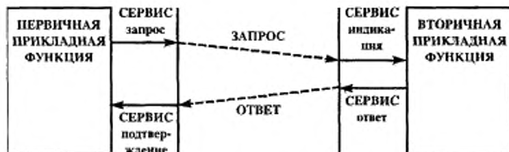
Рисунок 1 — Основные сервисы пользователя
