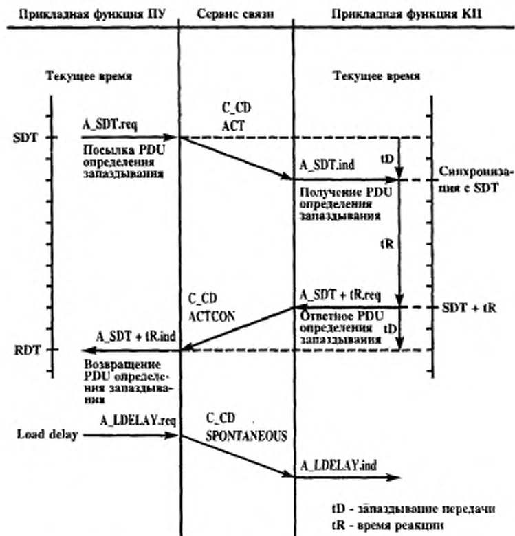
Рисунок 23 — Последовательная процедура — определение запаздывания передачи
