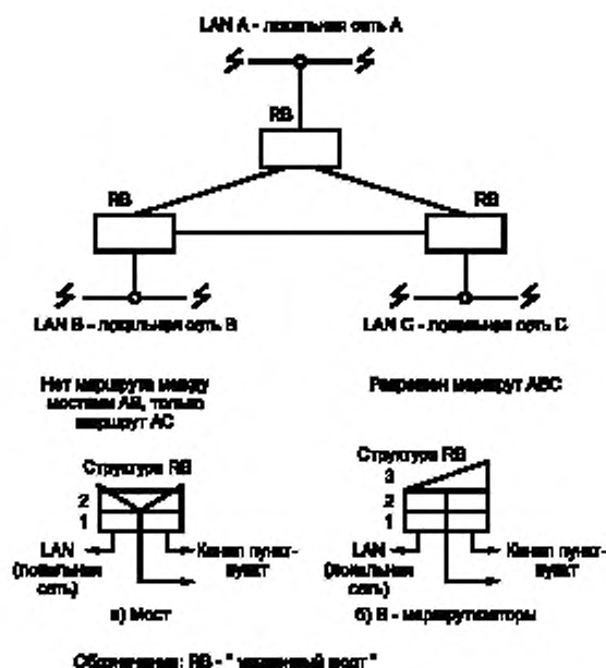
Рисунок 10 — Базовая структура с «удаленными мостами»
