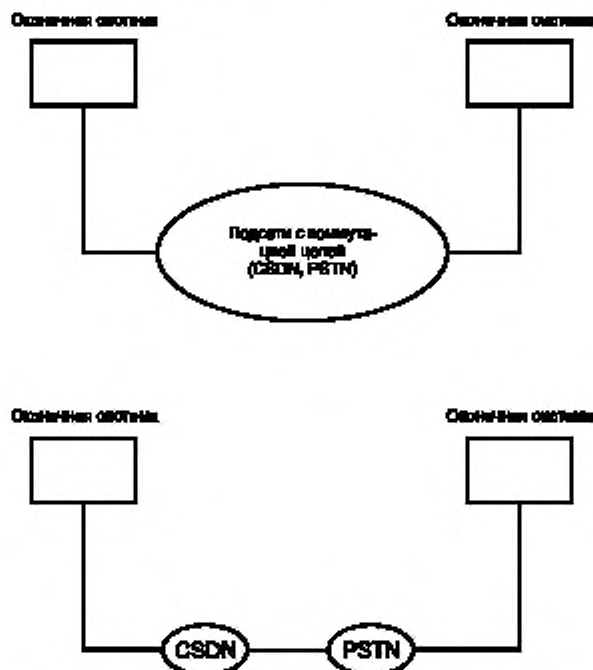
Рисунок 7 — Базовые структуры, основанные на коммутации цепей
