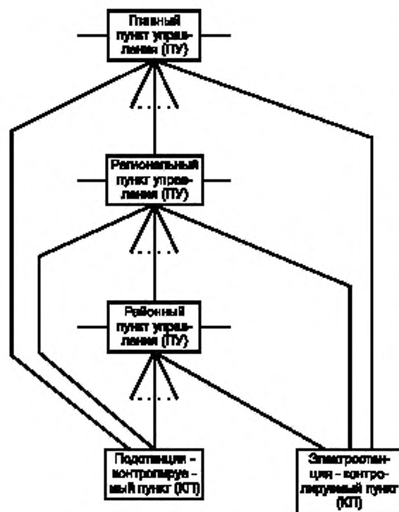
Рисунок 1 — Основная структура системы управления
