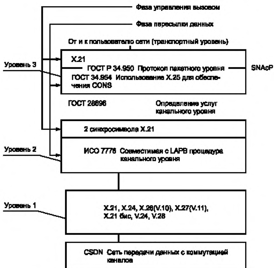
Рисунок 4 — Описание модели сети передачи данных с коммутацией каналов
