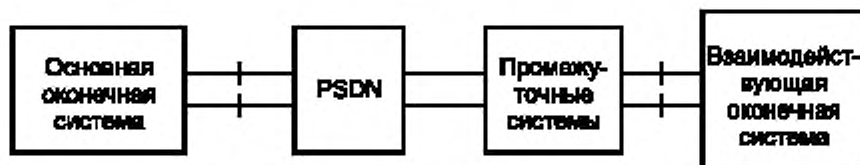
Рисунок 1 — Схема сети передачи данных с коммутацией пакетов
