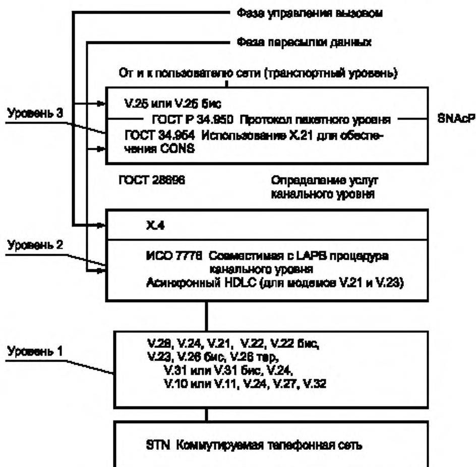
Рисунок 6 — Описание модели коммутируемой телефонной сети
