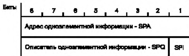
Рисунок 12 — Одноэлементная информация с адресом и описателем
