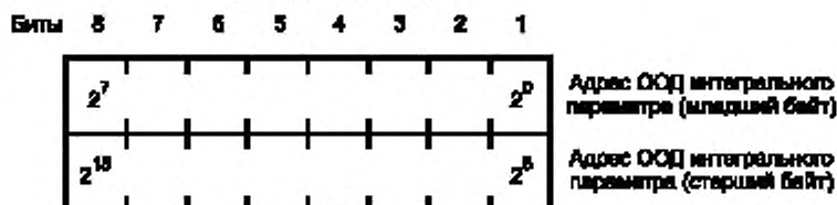
Рисунок 8 — Адрес ООД интегрального параметра (два байта)
