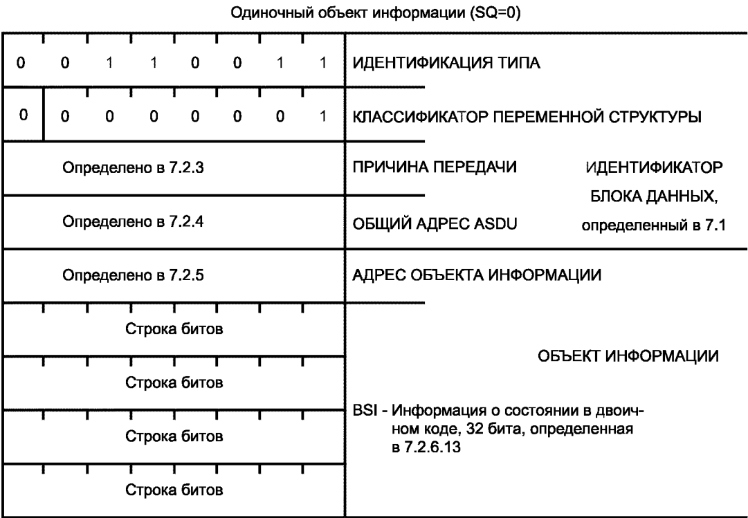
Рисунок 44 — ASDU. C_BO_NA_1. Строка из 32 битов
