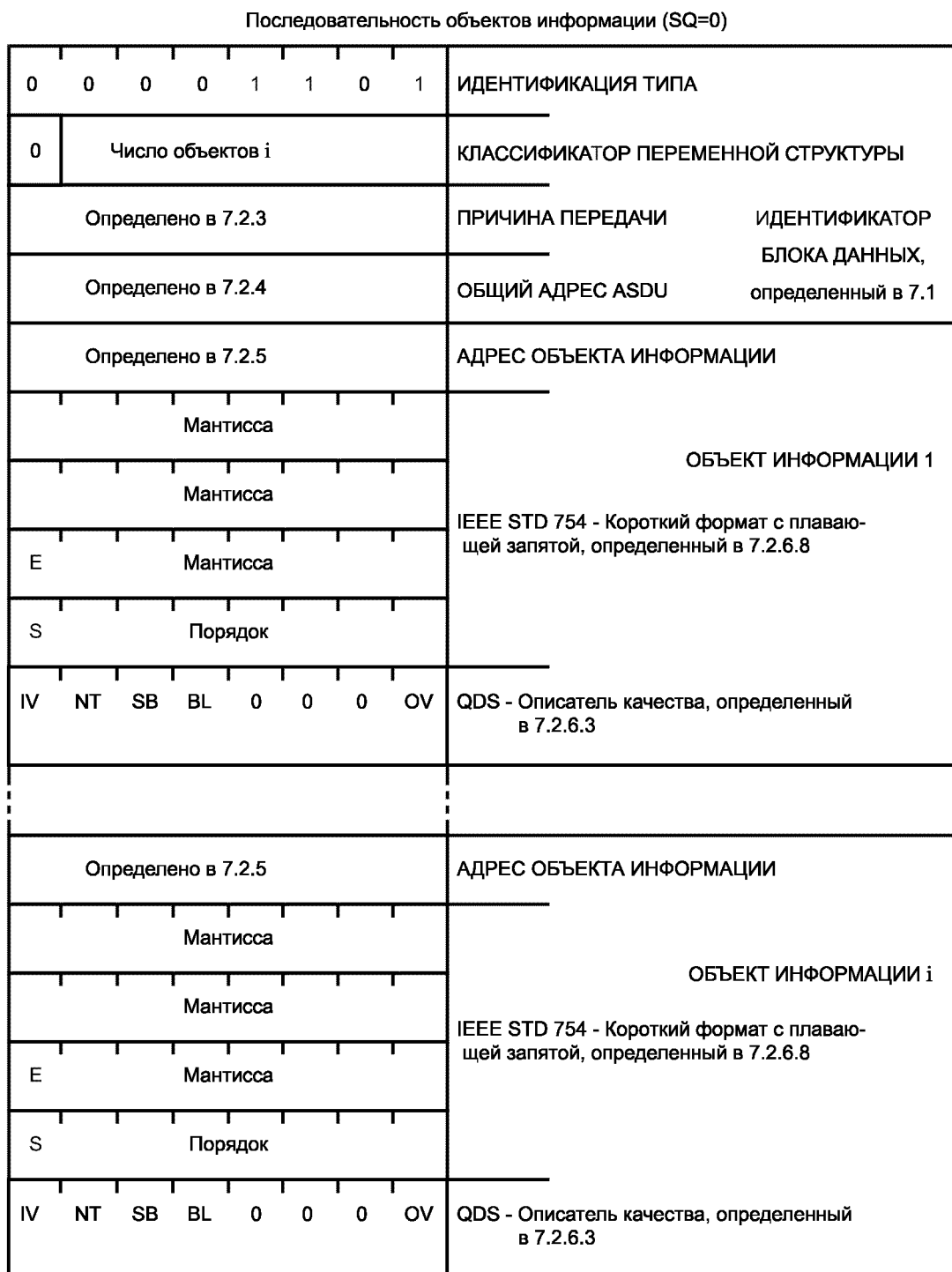
Рисунок 28 — ASDU. M_ME_NC_1. Значение измеряемой величины, короткий формат с плавающей запятой
