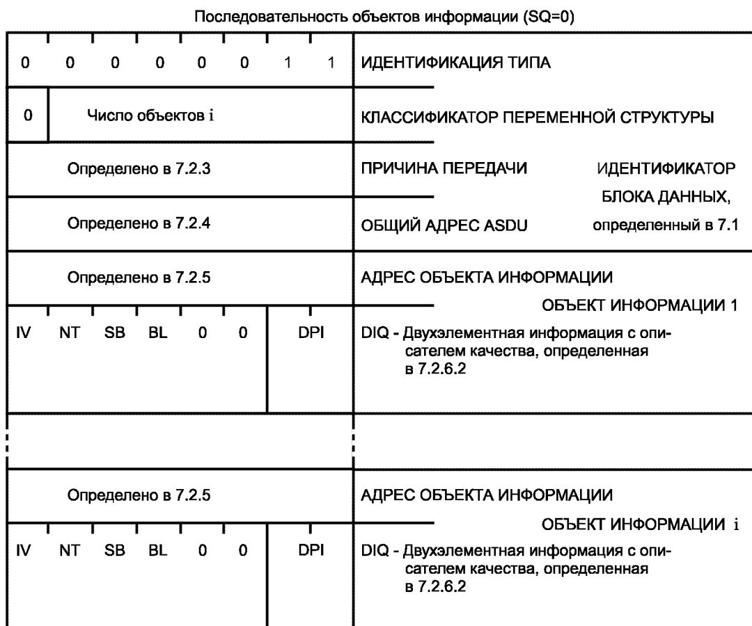
Рисунок 15 — ASDU. M_DP_NA_1. Двухэлементная информация без метки времени
