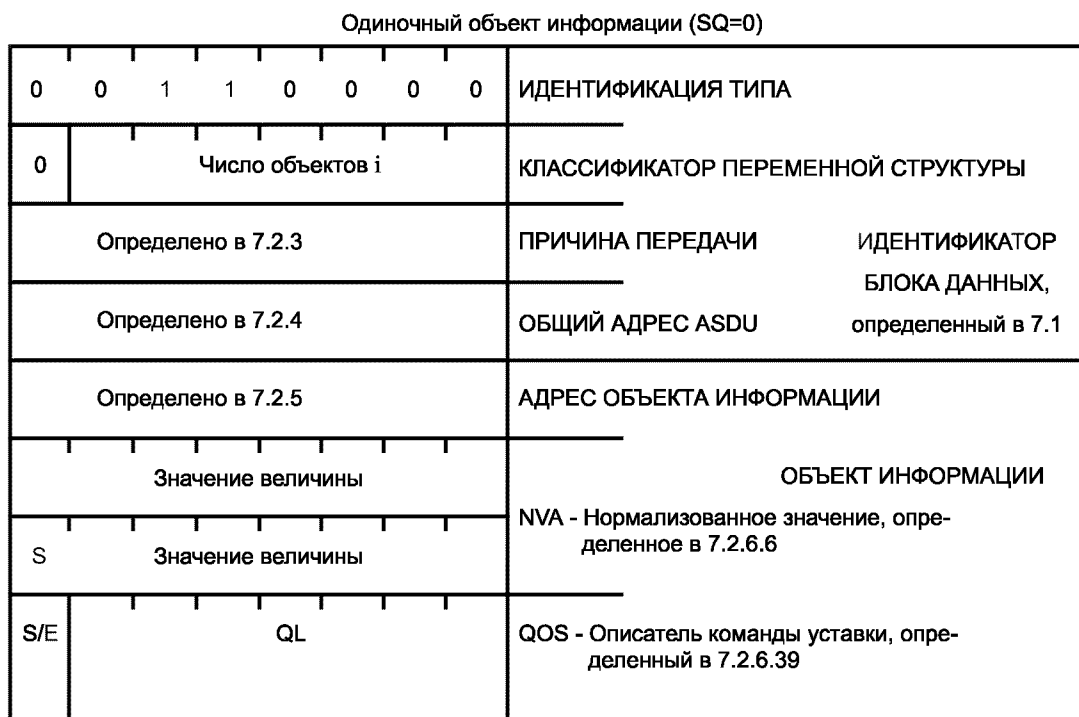
Рисунок 41 — ASDU. C_SE_NA_1. Команда уставки, нормализованное значение
