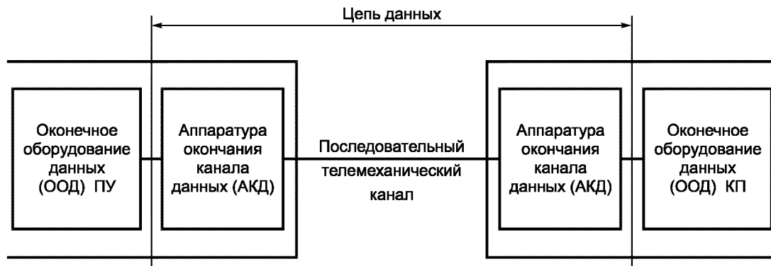
Рисунок 2 — Интерфейсы и соединения между ПУ и КП
