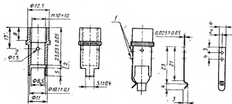
1 — заклепки или винты; 2 — отверстие Рисунок 5 — Корпус
