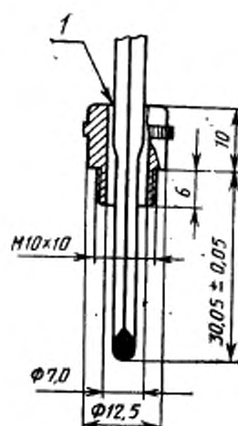
Рисунок 4 — Термометр и муфта
