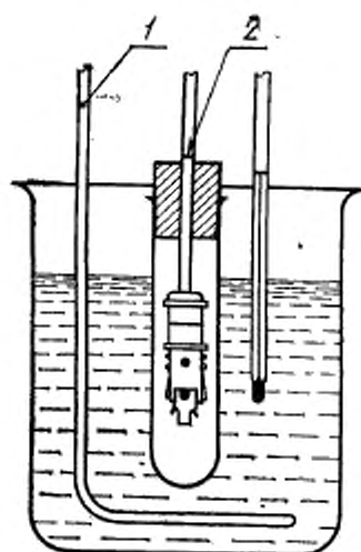
1 — мешалка; 2 — линия погружения
