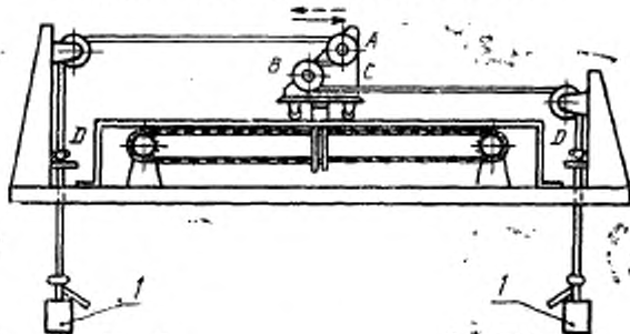
I — груз; A и B — шкивы; C — каретка; D — ограничительные зажимы
