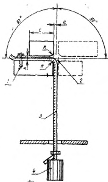
1 — узел крепления образца; 2 — ось изгиба; 3 — образец; 4 — груз
