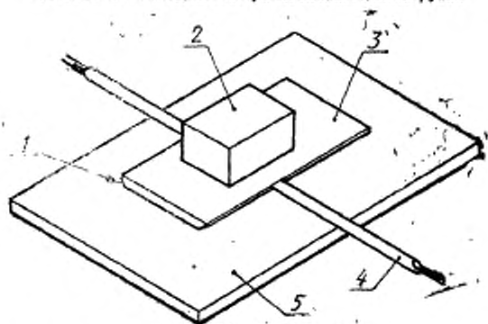
1 — радиус закругления; 2 — груз; 3 — подвижная пластина; 4 — образец кабеля; 5 — опорная пластина
