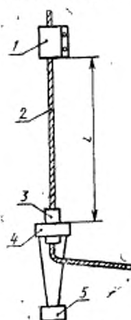
1 — неподвижный зажим; 2 — образец; 3 — концевая или зажимная муфта; 4 — вращающийся зажим; 5 — груз
