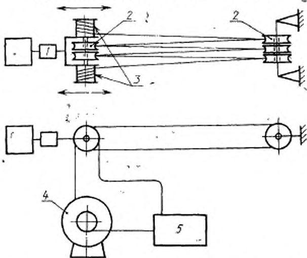
Оборудование для проведения испытания на растяжение
