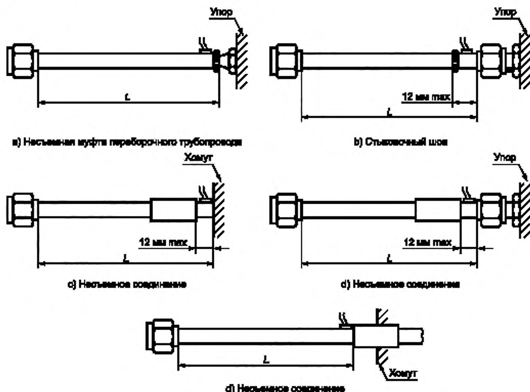
Рисунок 3 — Способы установки образцов с несъемной муфтой
