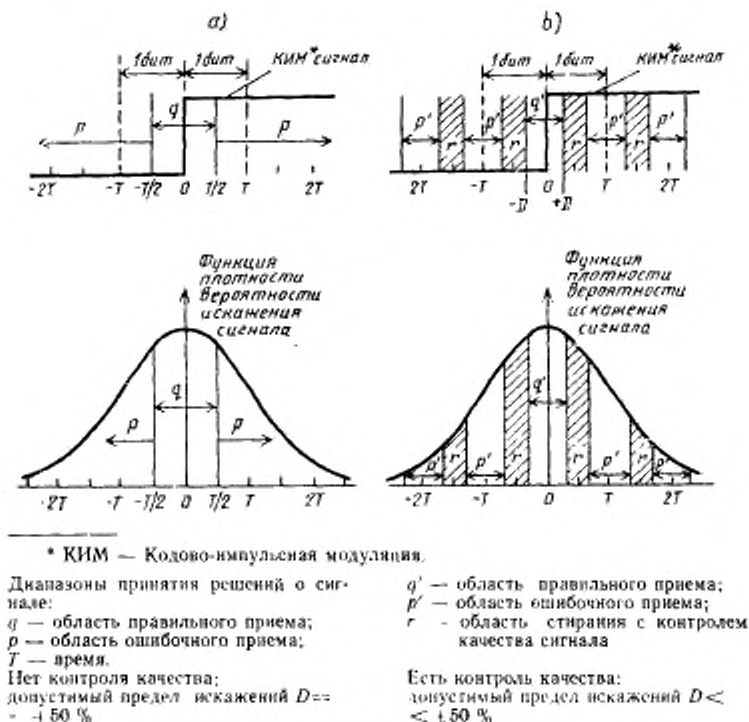
Рисунок А.1 — Обнаружение бита сигнала
