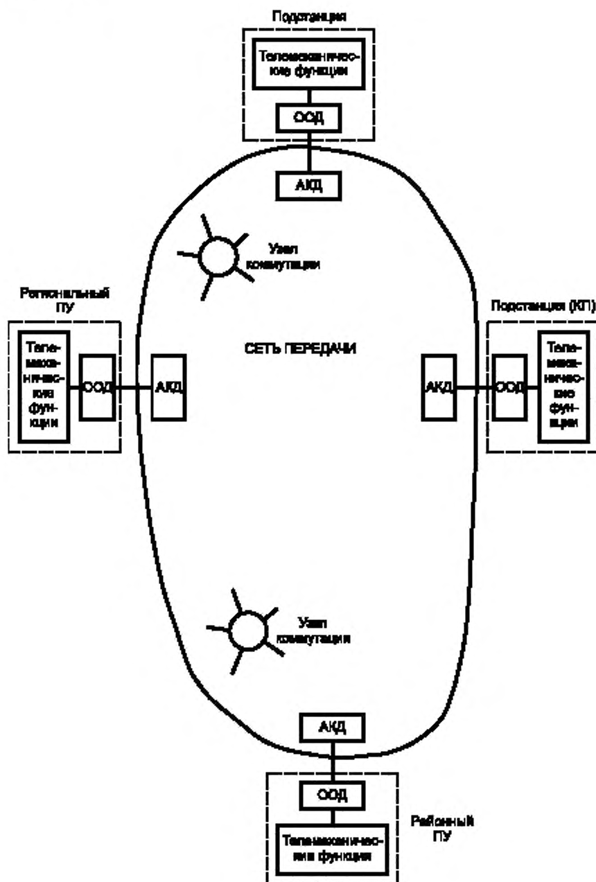
Рисунок 1 — Основная структура сети связи
