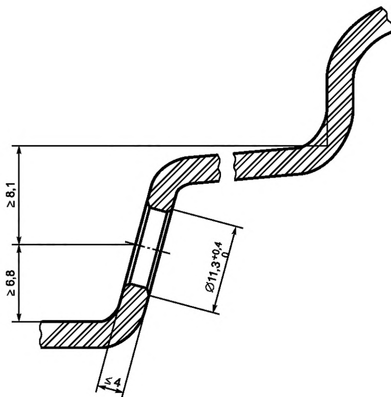
Рисунок 3 — Размеры вентиляльного отверстия для бескамерных шин
