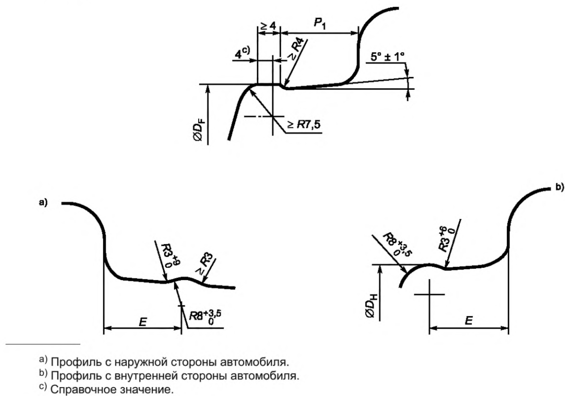
Рисунок 2 — Дополнительные исполнения профилей полок обода
