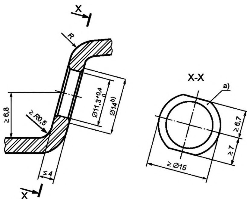
Рисунок 3 — Размеры вентиляльного отверстия для бескамерных шин
