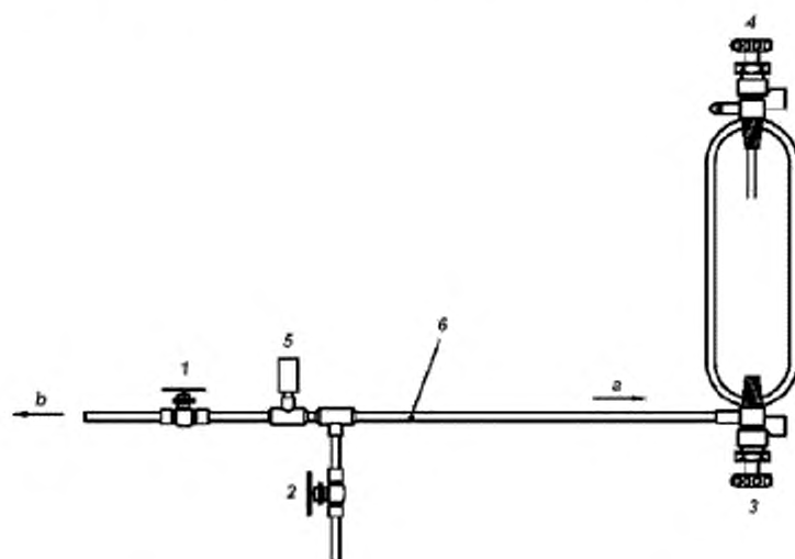
1 — регулирующий вентиль А; 2 — выпускной вентиль В; 3 — вентиль С; 4 — вентиль D; 5 — вентиль сброса давления; 6 — гибкая армированная трубка; а — к вентилу С; б — к вентилу на источнике с продуктом
