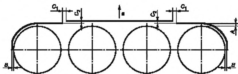
е) Несколько роторов, расположенных на одной линии
