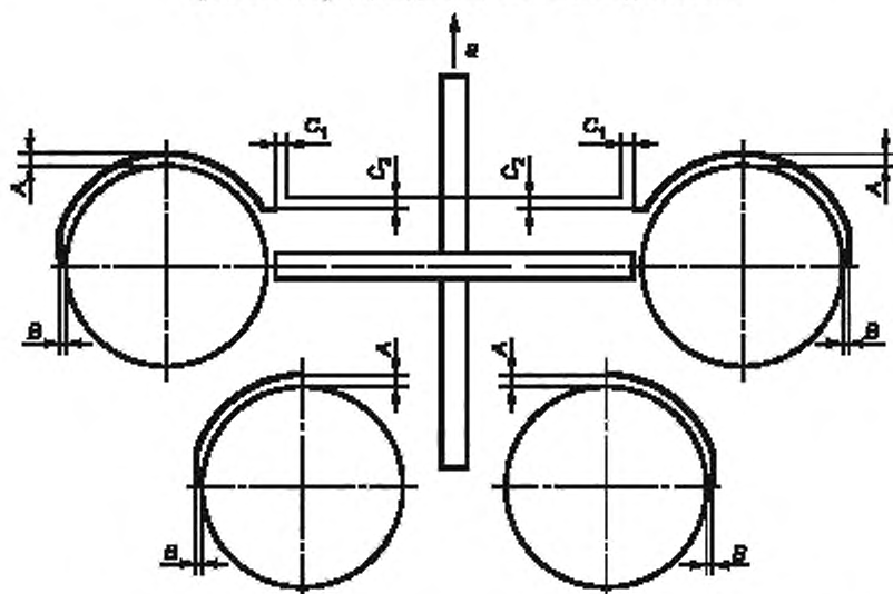
ж) Задние роторы, расположенные внутри относительно передних роторов
