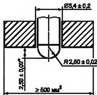
Рисунок 3 — Индентор для дюрометра типа АО
