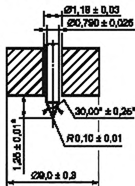
Рисунок 4 — Индентор для дюрометра типа АМ
