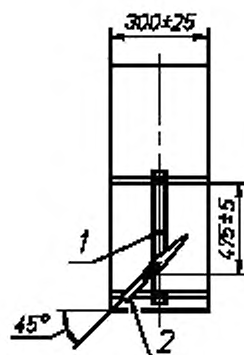
Рисунок 3 – Расположение горелки мощностью 1 кВт относительно образца
