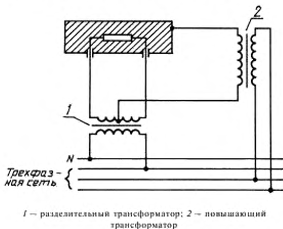
Рисунок 8 — Схема для испытания электрической прочности при рабочей температуре
