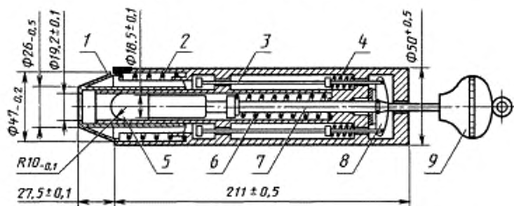
Устройство для испытания на удар
