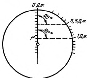
Рисунок 1.6 — Градуировка шкалы
