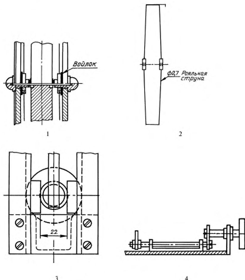
Рисунок 1.4 — Детали калибрующего устройства
