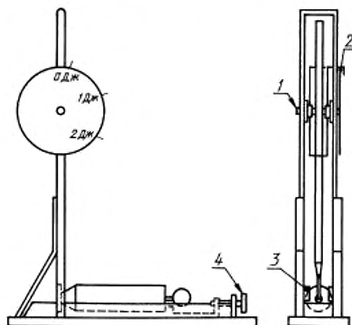
Рисунок 1.3 — Калибрующее устройство
