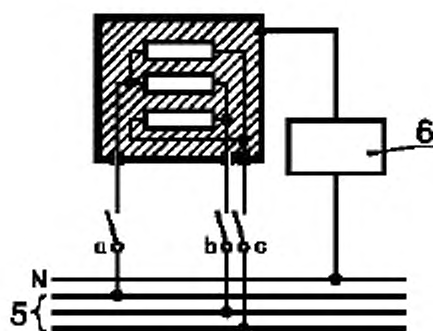
Рисунок 7 — Схема измерения тока утечки при рабочей температуре для трехфазных приборов, кроме приборов класса II
