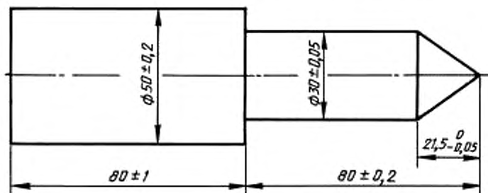
Рисунок 3 — Испытательный щуп
