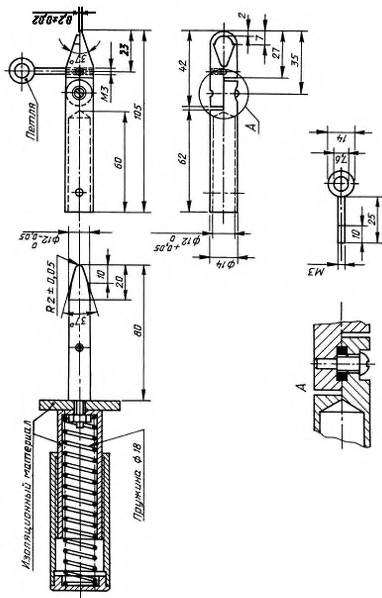
Рисунок 10 — Испытательный полупроводниковый палец
