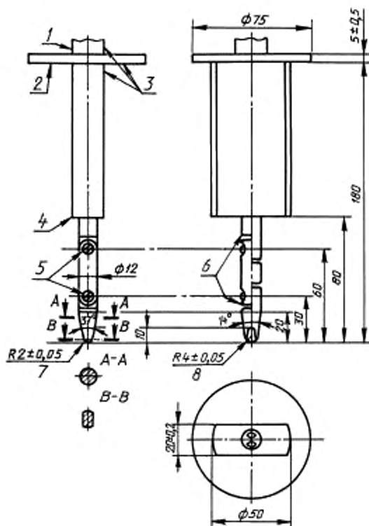
1 — ручка; 2 — ограждение; 3 — изоляционный материал; 4 — стопорная фланка; 5 — соединение; 6 — фланки (сняты на всех углах); 7 — цилиндрическая часть; 8 — сферическая часть
