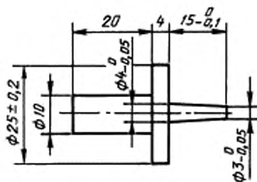
Рисунок 2 — Испытательный стержень
