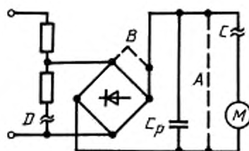
Параллельная цепь
