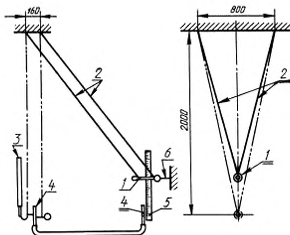
Рисунок 1.5 — Установка для настройки калибрующего устройства
