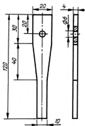
Рисунок 1.2 — Стальная пружина
