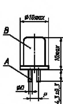
Размеры в миллиметрах
