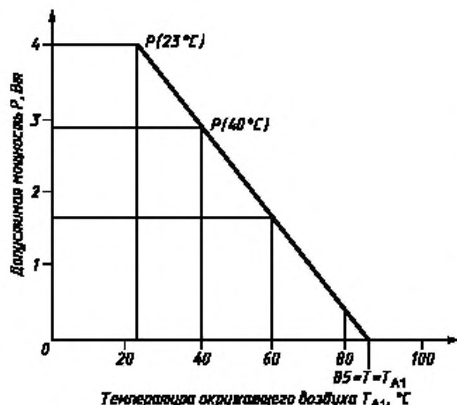
Рисунок 12 — Пример снижения мощности
