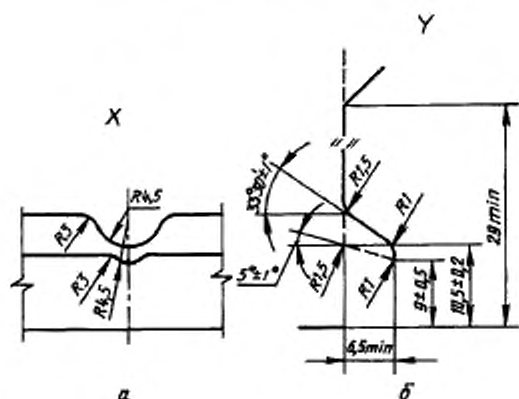
Деталь X — выемка
