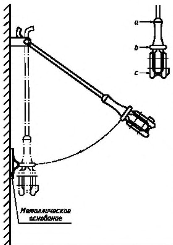
Рисунок 1 — Устройство для испытания светильника на удар
