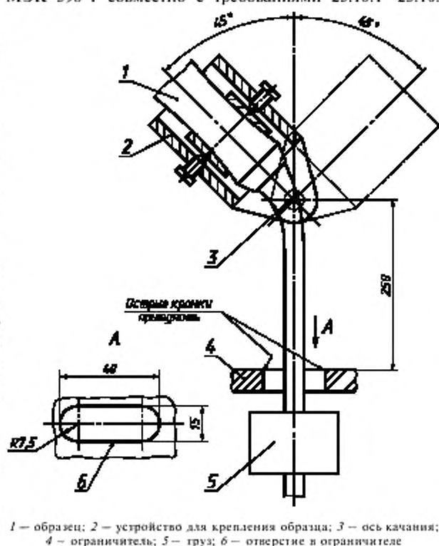
Рисунок 2 — Устройство для испытания светильника на изгиб
