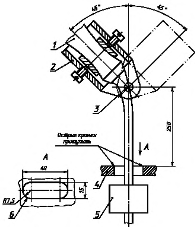
1 — образец; 2 — устройство для крепления образца; 3 — ось качения; 4 — ограничитель; 5 — груз; 6 — отверстие в ограничителе
