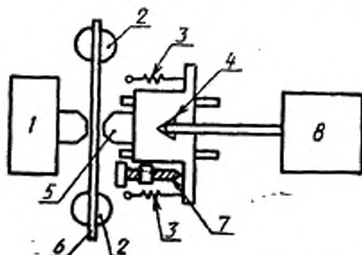
1 — неподвижный контакт; 2 — держатель образца; 3 — пружина; 4 — шуп; 5 — контакт на прецизионной платформе; 6 — образец; 7 — микрометрический винт; 8 — электронный микрометр
