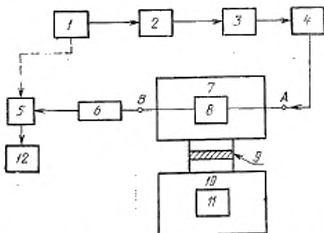
1 — модулированный источник света; 2 — оптические фильтры (монокроматор); 3 — имитатор ввода на входе; 4 — устройство выделения мод оболочки; 5 — синхронный детектор; 6 — оптический детектор; 7 — камера с регулируемой температурой; 8 — испытываемый образец; 9 — затвор; 10 — экранированная камера; 11 — источник гамма-излучения; 12 — регистрирующее устройство.
