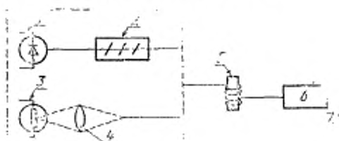
Аппаратура для измерения затухания на установленной длине волны
