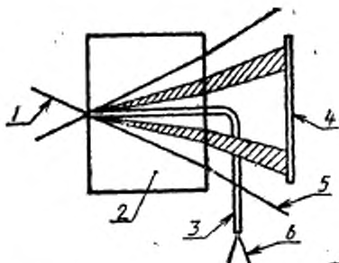
Метод преломления в ближнем поле. Схема
