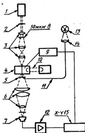
1 — лазер; 2 — четвертьволновая пластинка; 3 — линза; 4 — ячейка с жидкостью; 5 — диск; 6 — линза; 7 — фотодиод; 8 — точечное отверстие, 50 мкм; 9 — электронный микрометр; 10 — датчик; 11 — волокно; 12 — усилитель; 13 — линза; 14 — линза; 15 — двухкоординатный самописец
