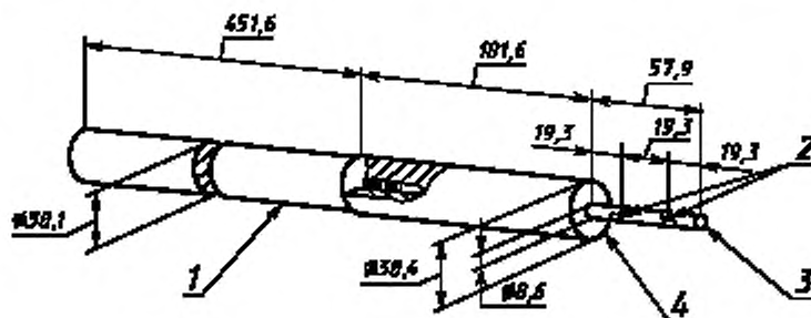
1 – ручка; 2 – точки соединения; 3 – сфера радиусом 4,3 мм; 4 – стопорная фаска
