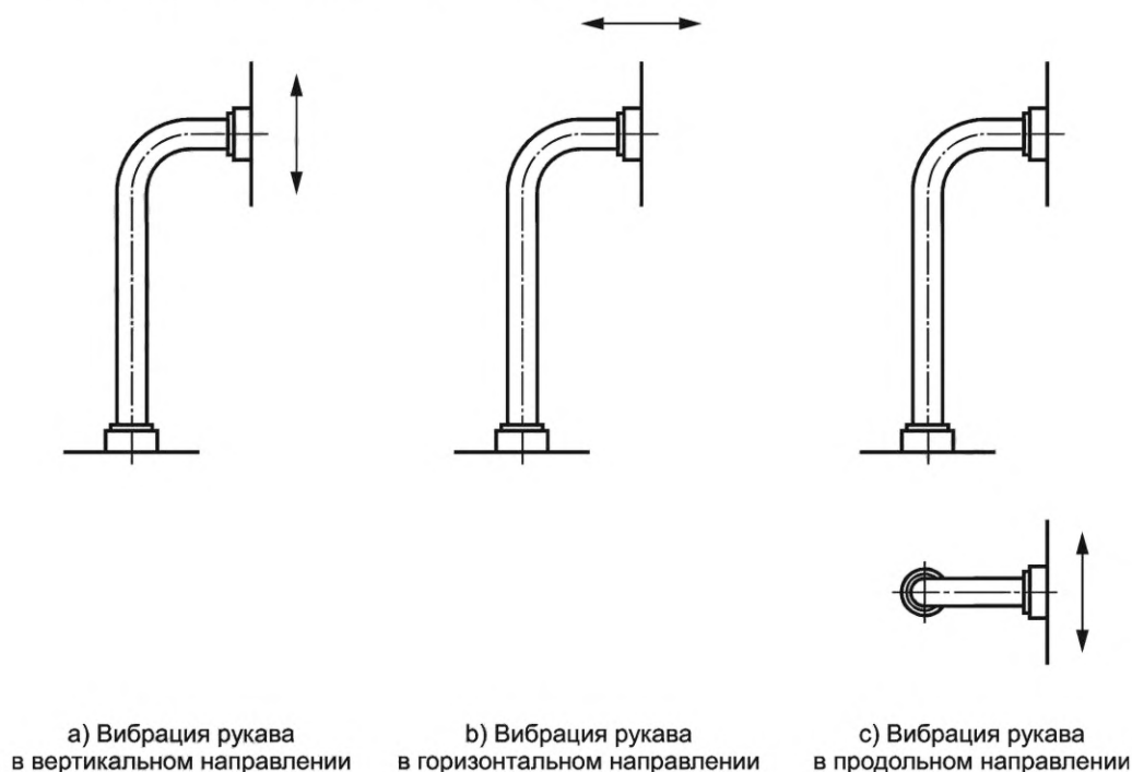
Рисунок С.1 — Направления вибрации испытываемого образца
