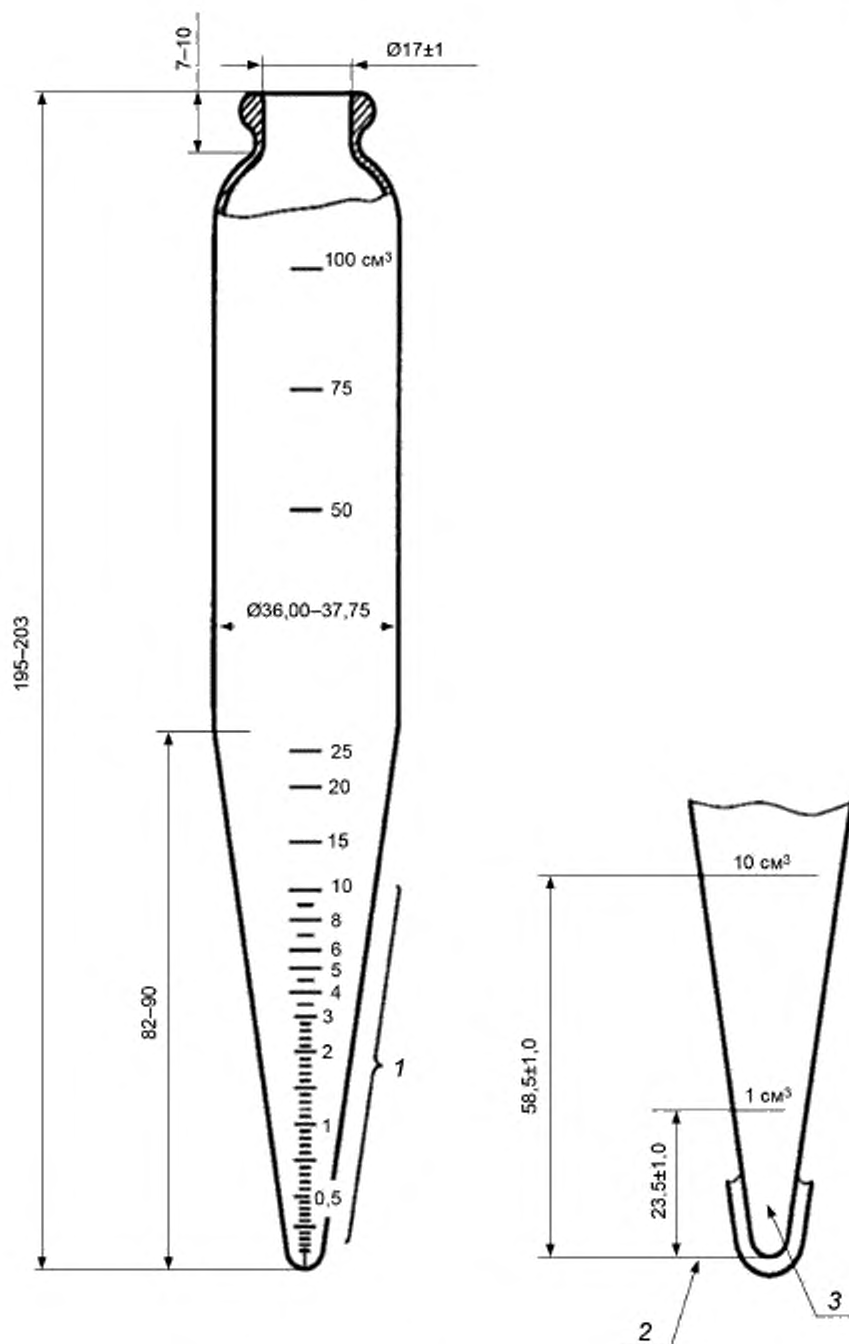
1 — стенка конуса (должна быть прямой); 2 — уровень внутренней поверхности дна, 3 — очертания (форма) внутренней поверхности конуса
