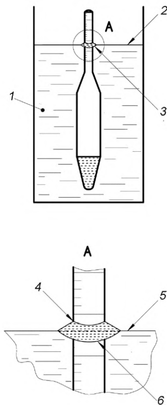
1 — жидкость; 2 — горизонтальная плоская поверхность жидкости; 3 — нижняя часть мениска; 4 — место считывания шкалы; 5 — горизонтальная плоская поверхность жидкости; 6 — мениск
