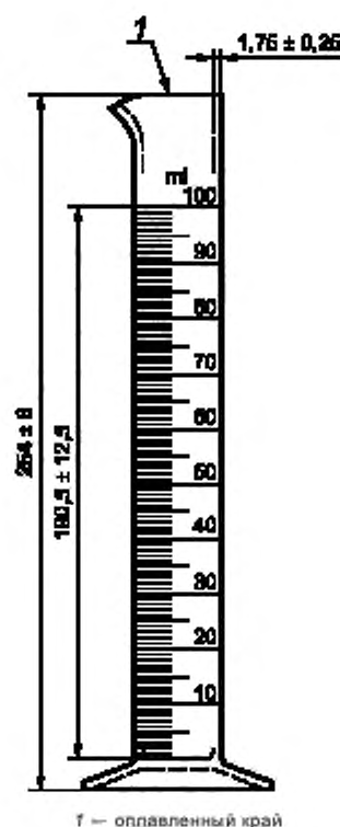
Рисунок 5 — Приемный цилиндр вместимостью (100,0 \pm 1,0) мл
