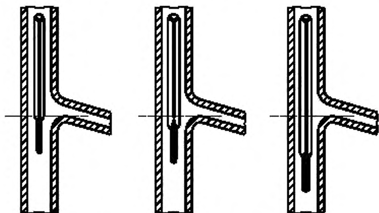
Рисунок 8 — Положение термометра в колбе для разгонки
