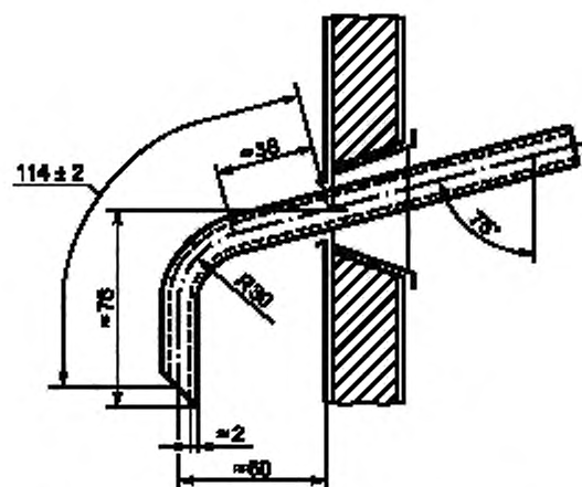
Рисунок 4 — Нижний конец трубки холодильника
