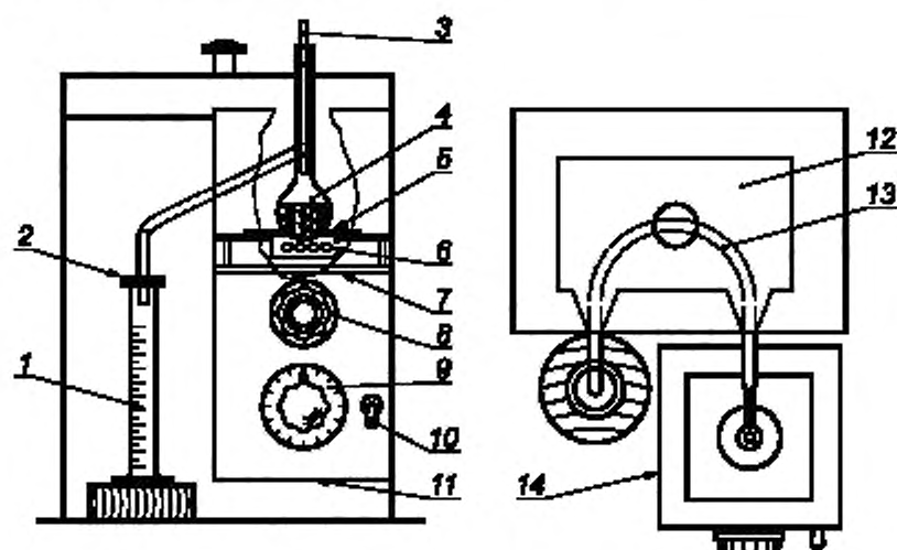
Рисунок 1 — Аппарат в сборе с газовой горелкой
