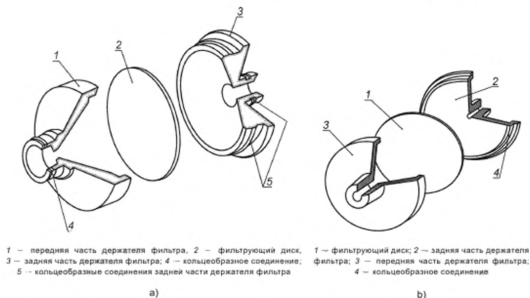
Рисунок 4 — Схема повушки для дыма с фильтрующим диском из стекловолокна
