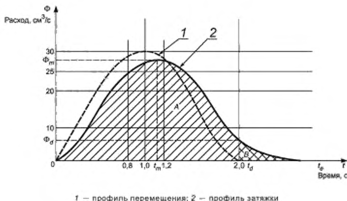
Рисунок С.1 — Схематическое изображение профиля затяжки сигареты
