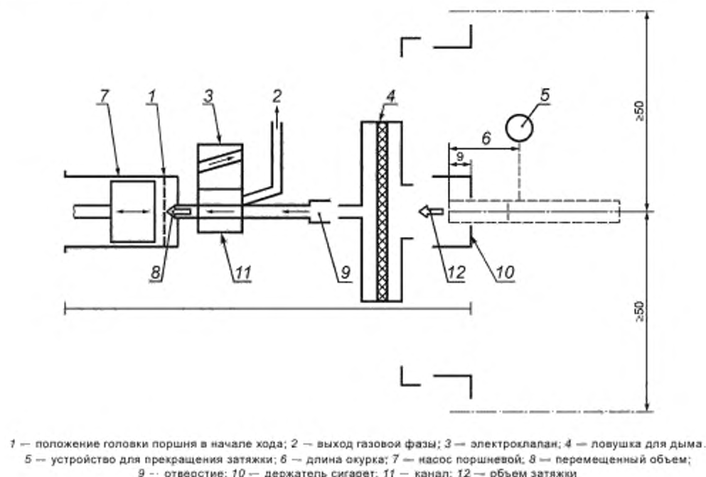
Рисунок 3 — Схема работы курительной машины
