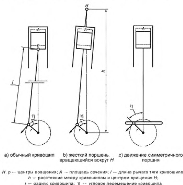
Рисунок В.1 — Пример конструкции механизма поршень/кривошип
