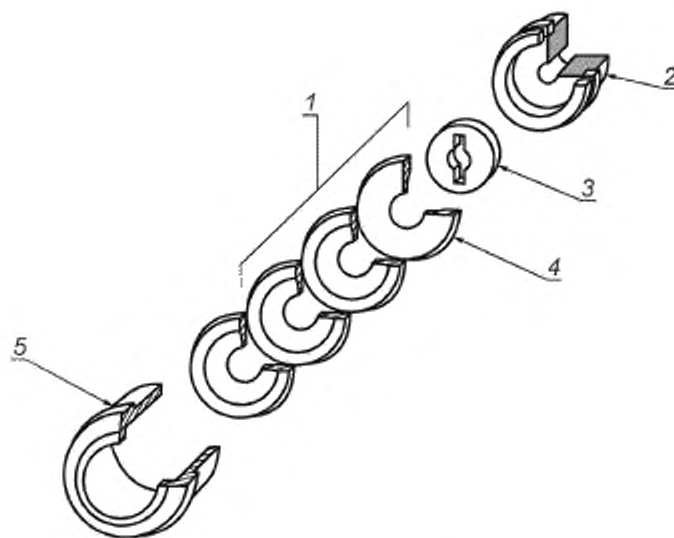
1 — лабиринтовые уплотнения, 2 — опора перфорированного диска, 3 — перфорированный диск; 4 — задняя часть лабиринтового соединения, 5 — колпачок для лабиринтового соединения
