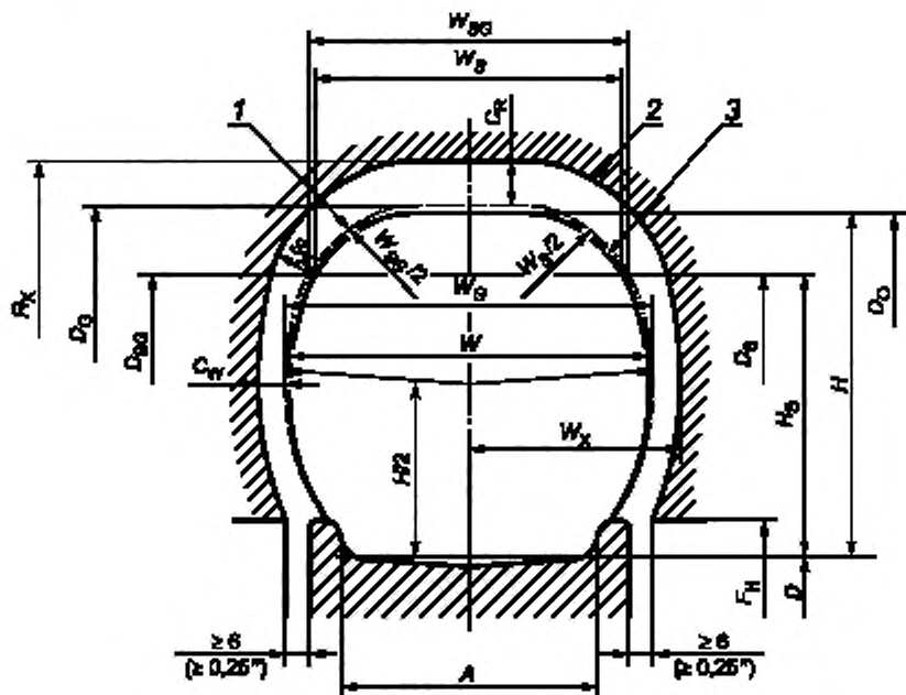
Рисунок 2 — Допуски на увеличение и на зазоры
