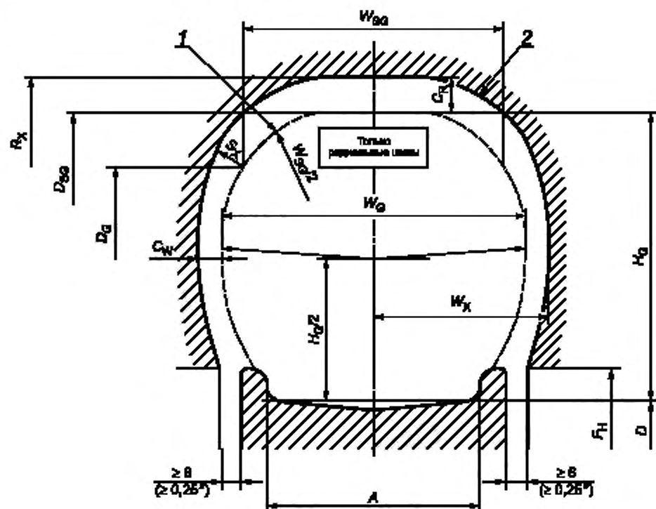
b — Допуски на увеличение и зазоры для радиальных шин
