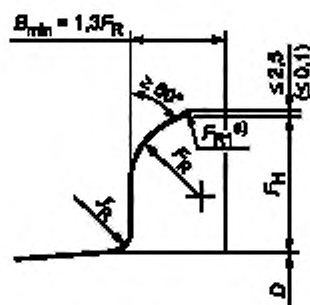
Рисунок 8 — Увеличение высоты бортовой закраины от установленного размера
