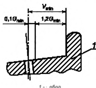
Рисунок 9 — Расположение отверстия для вентиля камерной шины
