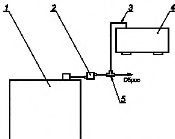
Рисунок Б.1 — Газовая схема для подачи ГС от генератора со встроенным побудителем расхода на газоанализатор-компаратор
