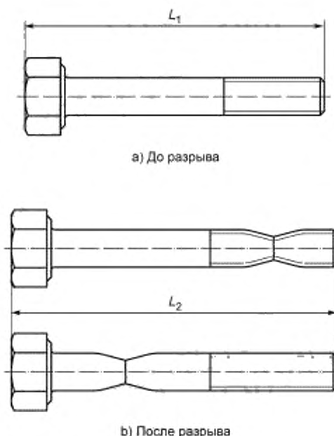
Рисунок 8 — Определение удлинения после разрыва A
