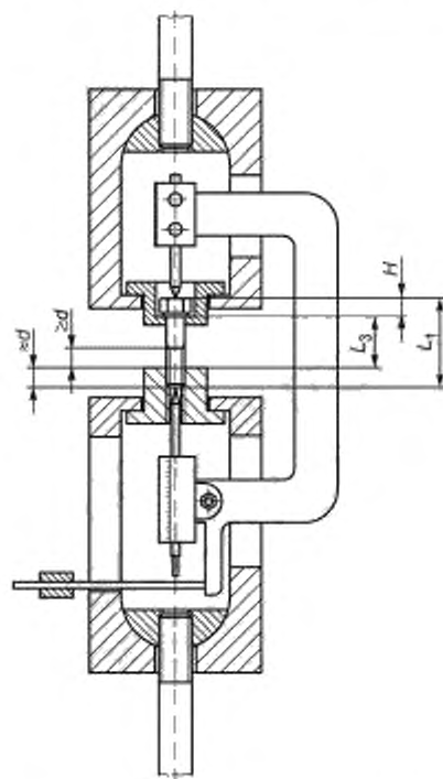
Рисунок 6 — Тензометр, установленный на болт в самоцентрирующих зажимах
