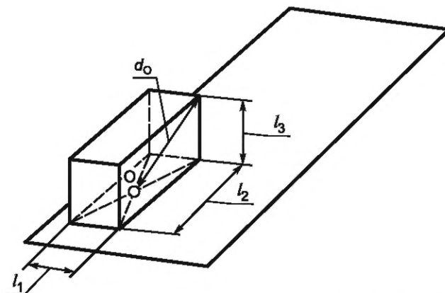
а) Одна звукоотражающая плоскость, d_O = \sqrt{(l_1/2)^2 + (l_2/2)^2 + l_3^2}
