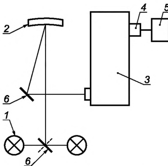
Рисунок 2 — Блок-схема установки для измерения СПЭЯ
