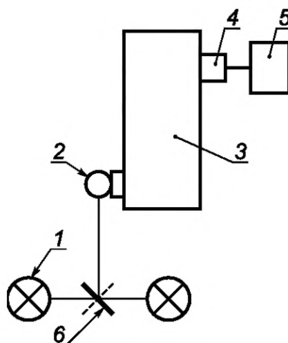
Рисунок 1 — Блок-схема установки для измерения СПЭО
