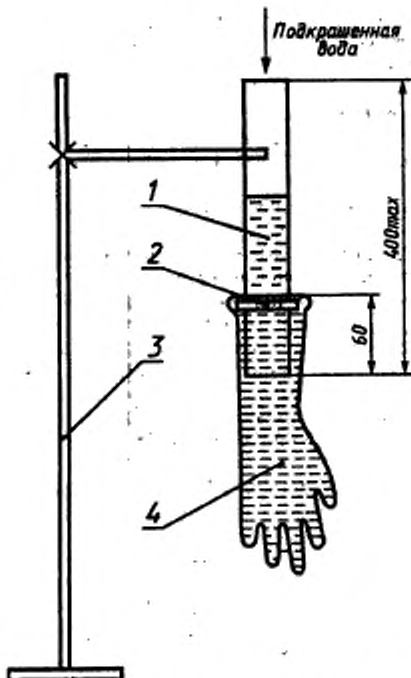
1 — цилиндр; 2 — муфта; 3 — опорная стойка; 4 — испытываемая перчатка
