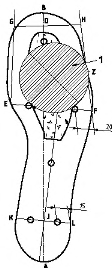
Рисунок D.1 — Измерение удельного электрического сопротивления
