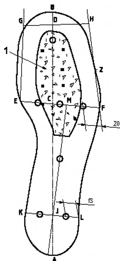
О – позиция потайных заклепок; 1 – нержавеющая сталь Рисунок А.1 — Рисунок несъемной стельки
