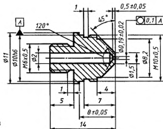
Рисунок А.2 — Схема газовой форсунки
