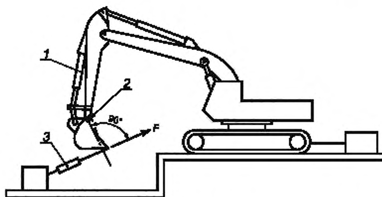
а) Гидравлический экскаватор с ковшом «обратная лопата»
