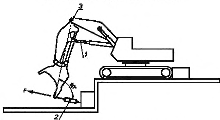
б) Гидравлический экскаватор с ковшом «прямая лопата»
