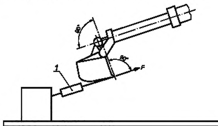
Рисунок 2 — Типовая схема измерения максимального усилия, развиваемого гидроцилиндром ковша (см. 4.8.3)
