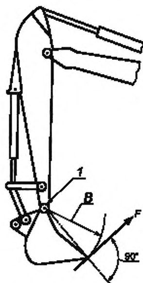
а) Оборудование «обратная лопата»
