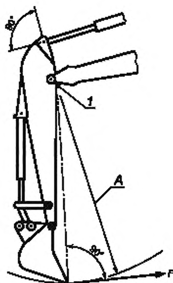
а) Оборудование «обратная лопата»
