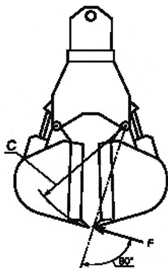
Рисунок 7 — Рабочий орган захват (рейфер). Расчет усилия замыкания (см. 5.2.4)
