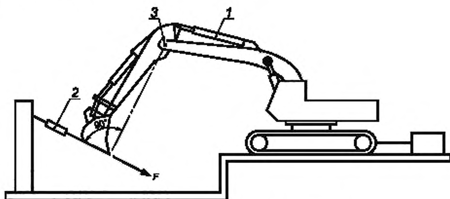
а) Гидравлический экскаватор с ковшом «обратная лопата»
