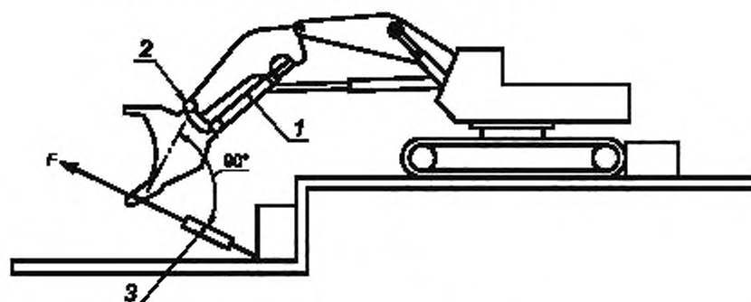
б) Гидравлический экскаватор с ковшом «прямая лопата»
