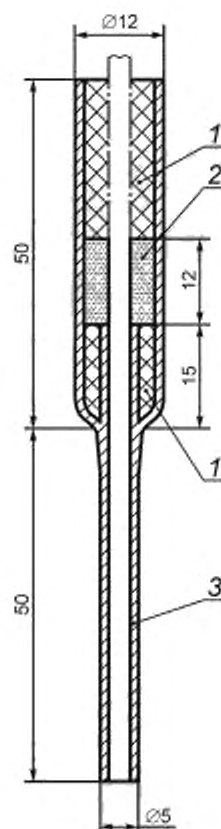
Рисунок 3 — Влагонепроницаемая втулка В
