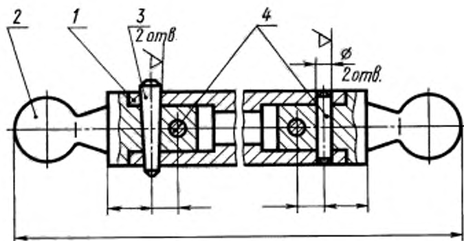
Сборочный чертеж
