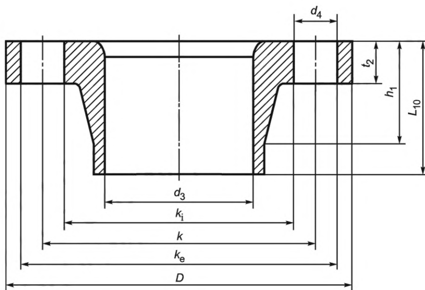
Рисунок 6 — Размеры фланцевой втулки
