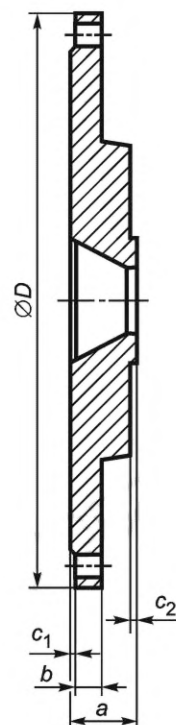
Рисунок 27 — Переходной фланец PN 40
