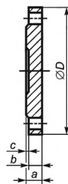
Рисунок 21 — Глухой фланец PN 16
