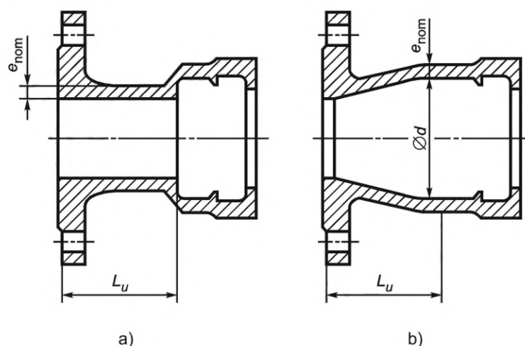
Рисунок 5 — Фланцевый раструб
