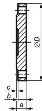
Рисунок 23 — Глухой фланец PN 40
