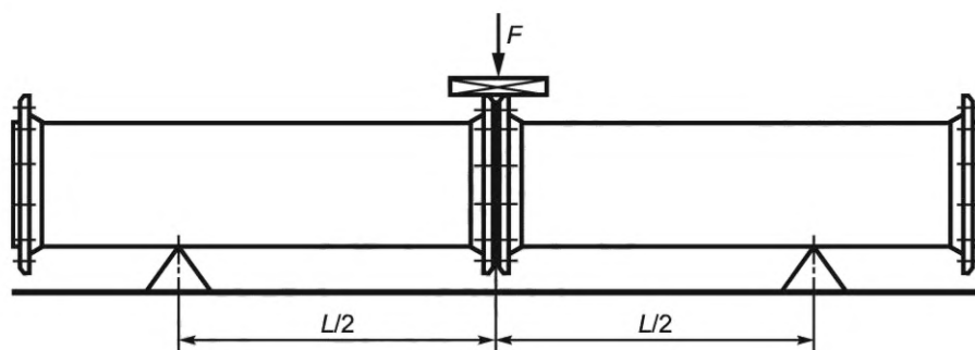
Рисунок 3 — Испытание на прочность и герметичность фланцевых соединений
