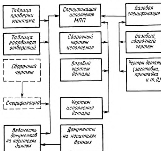
Пример построения комплекта конструкторских документов для МПП
