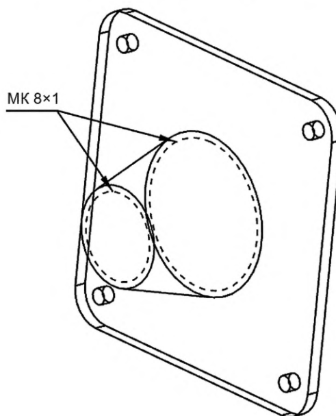
Рисунок 3 — Примеры обозначения конической резьбы
