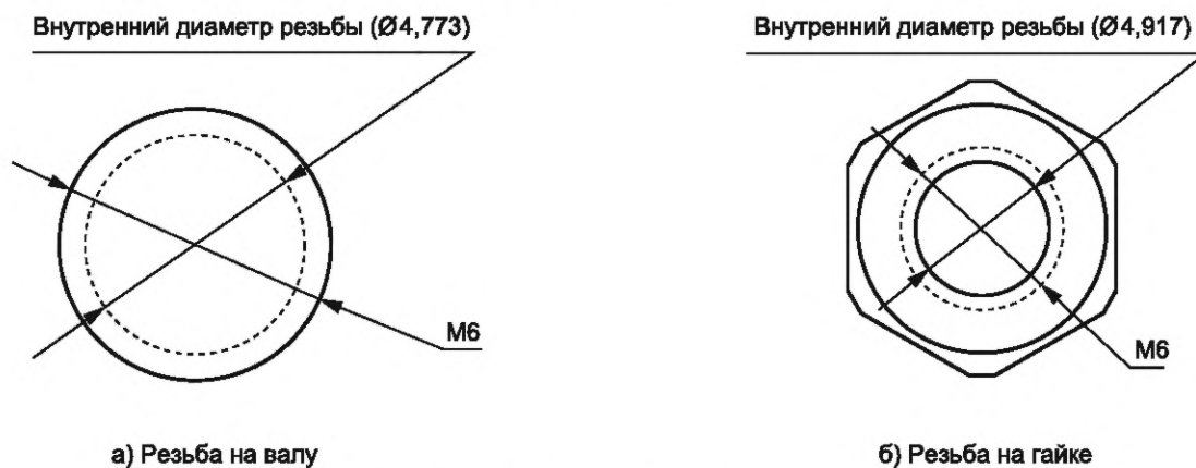
Рисунок 2 — Примеры ЭМД с резьбой М6 согласно ГОСТ 24705
